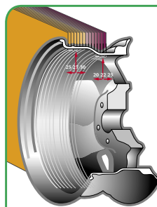
Programme Plans Mobiles "Shift Plane" (en Alu P) pour utilisation de masses multiples de cinq grammes, disponibles sans nécessité de coupes partielles (Brevet Corghi)
